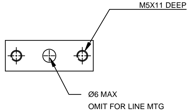
SUBPLATE DIMENSION
